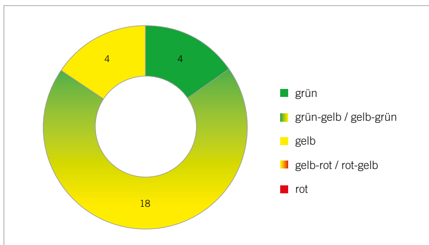
Abbildung 1. Q+Ampel-Statistik Studienjahr 2018
